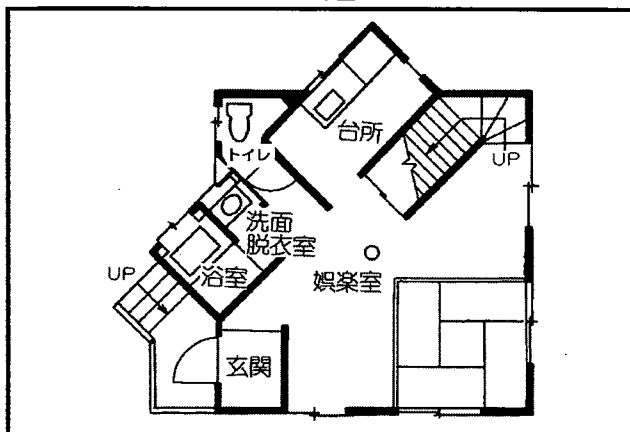
1階
